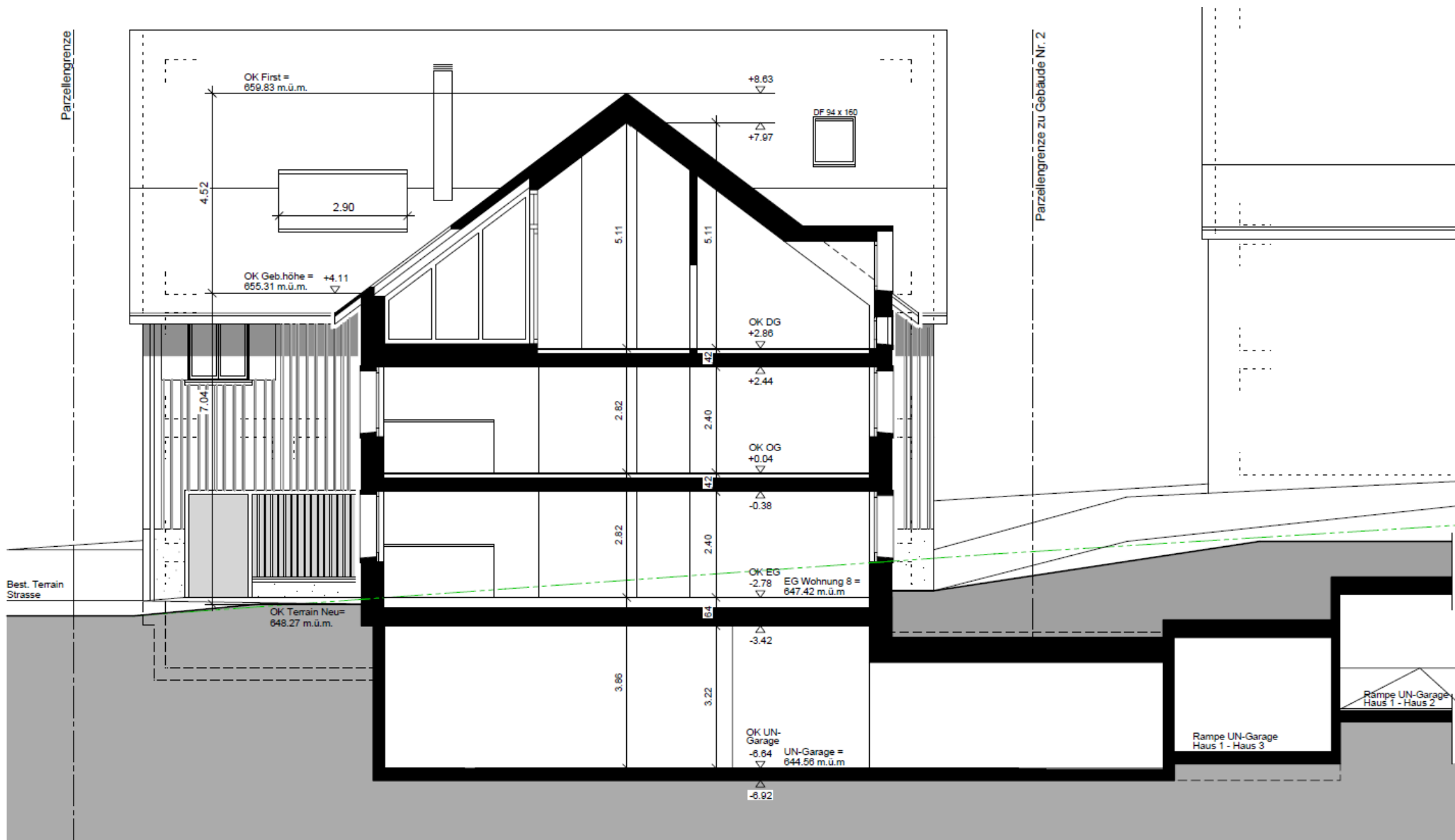
SCHNITT 2 - 2
