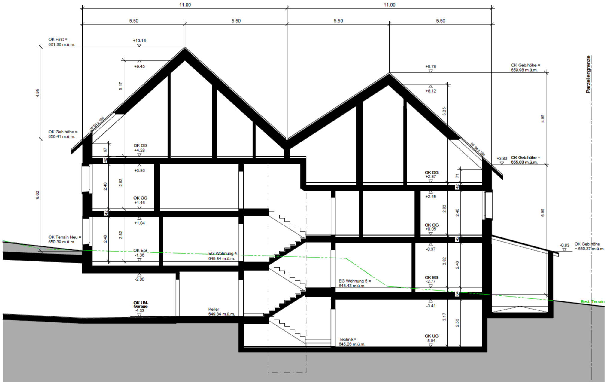
SCHNITT 1 - 1
