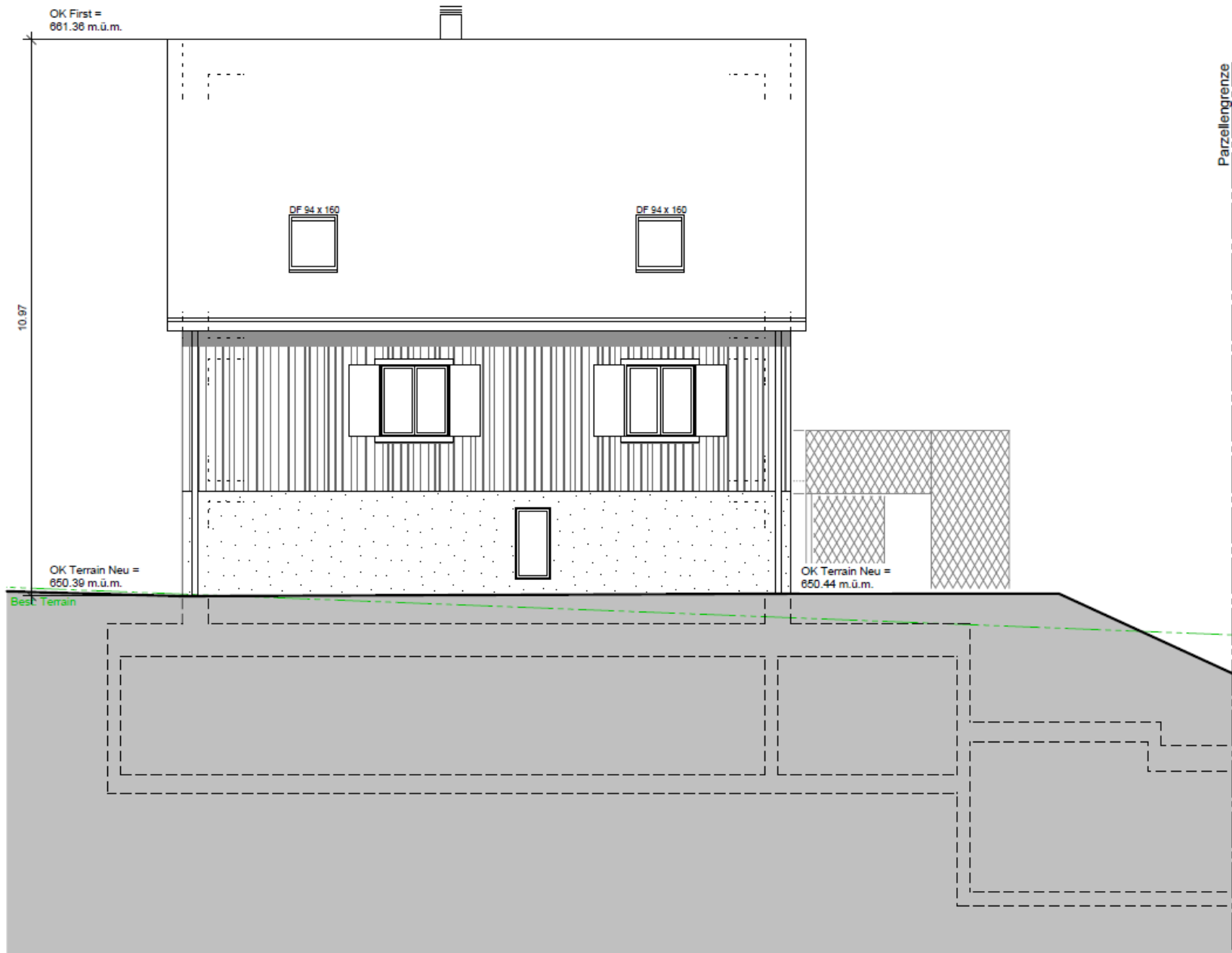
ANSICHT WESTFASDADE
