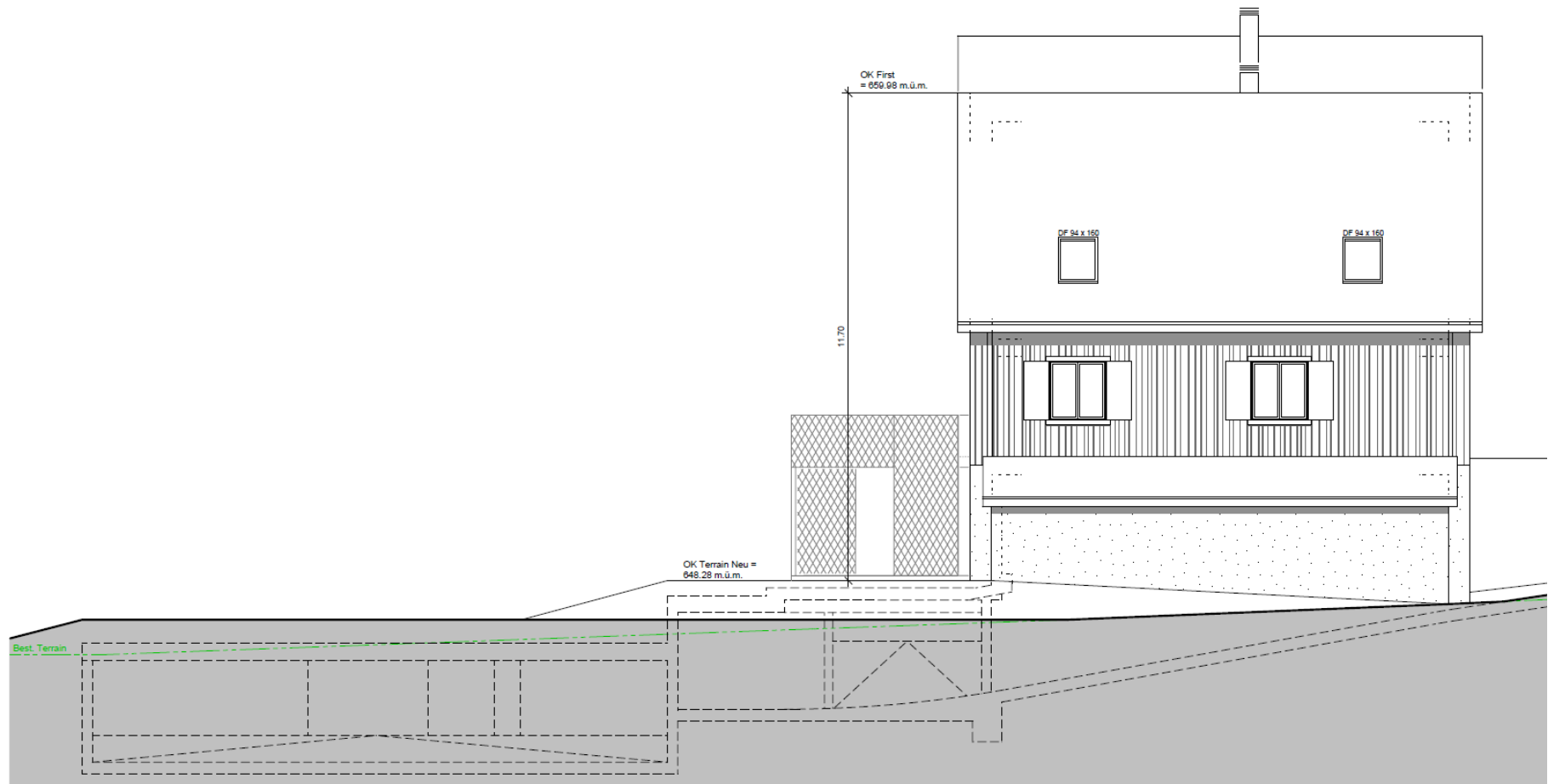
ANSICHT OSTFASSADE
